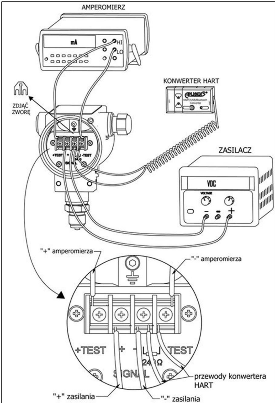
Rys.1. Wizualny układ podłączenia przetwornika do pętli prądowej w celu przeprowadzenia testu sprawdzającego.
